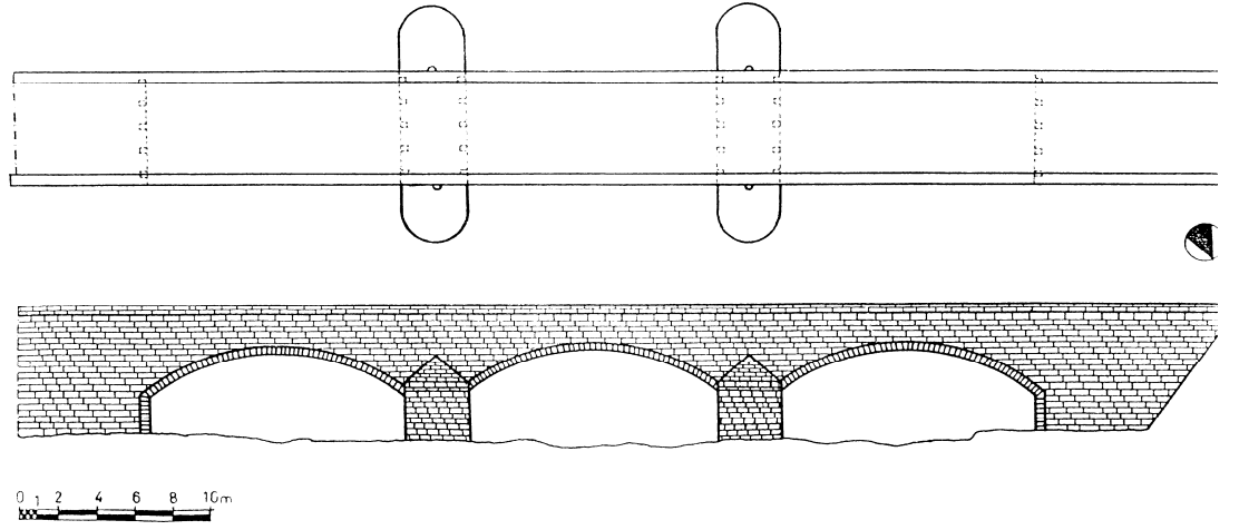
Figür 17- Berta Köprüsü Planı ( Aytekin 1999, 261, Çizim:75 )
