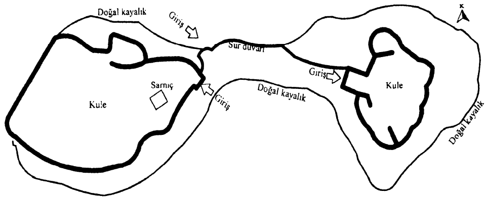
Figür 70-Oltu/Iğdeli Kalesi Plan Krokisi, (Gündoğdu et al 2002,39, Çizim:9)
